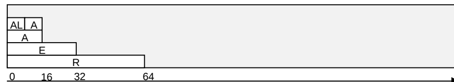
Рис. 2. Фрагмент адресного пространства регистров Intel 64.
