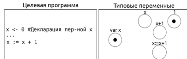
Рис. 1. Фрагмент анализируемой программы на языке Self (слева) и созданные для него типовые переменные (справа). Типовая переменная для декларации x помечена как var x , чтобы отличать её от выражения x (операнда сложения).
