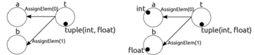
Рис. 10. Связи вида AssignElem , создаваемые при анализе присваивания списку переменных, например: a, b = t . Слева показаны типовые переменные до пропации типов по соответствующим рёбрам, справа — после.
