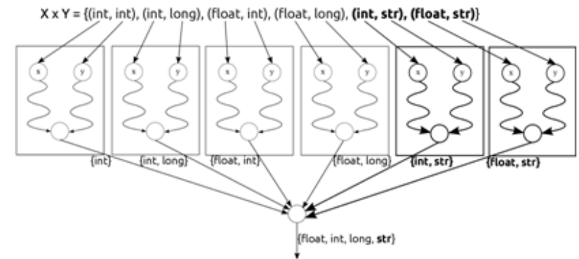
Рис. 6. АДП для вызова \max(x, y) , где X = \text{type}(x) = \{\text{int}, \text{float}\} , Y = \text{type}(y) = \{\text{int}, \text{long}, \text{str}\} . Здесь показано, что происходит при расширении типа аргумента вызова. Жирным шрифтом выделены «новые» структуры, создаваемые во время повторного вычисления декартова произведения.
