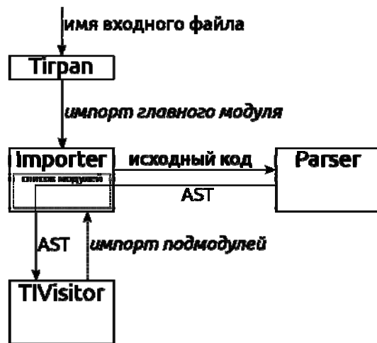
Рис. 7. Общая схема работы программы.
