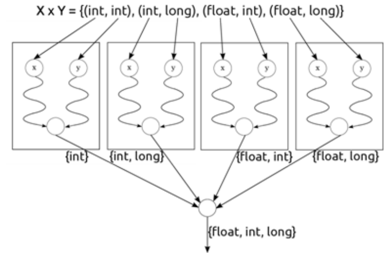
Рис. 5. АДП для вызова \max(x, y) , где X = \text{type}(x) = \{\text{int}, \text{float}\} , Y = \text{type}(y) = \{\text{int}, \text{long}\} .
